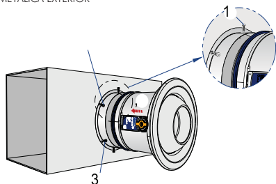
EXECUÇÃO COM ACESSÓRIO DE MONTAGEM A CONDUITA RECTANGULAR: TJN-K SEM FORRA METÁLICA EXTERIOR
