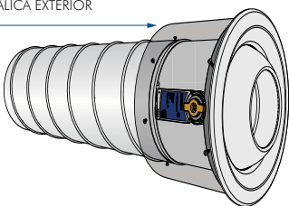
EXECUÇÃO COM ACESSÓRIO DE MONTAGEM A CONDUITA RECTANGULAR: TJN-K SEM FORRA METÁLICA EXTERIOR
