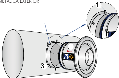
EXECUÇÃO COM ACESSÓRIO DE MONTAGEM A CONDUITA REDONDA: TJN-R SEM FORRA METÁLICA EXTERIOR
